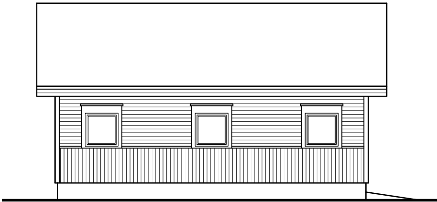
JULKISIVU LUOTEESEEN
