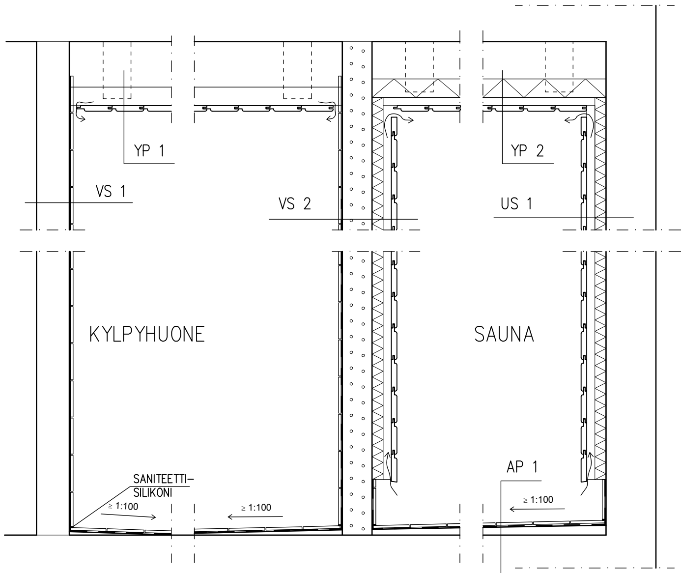
LEIKKAUS A-A
